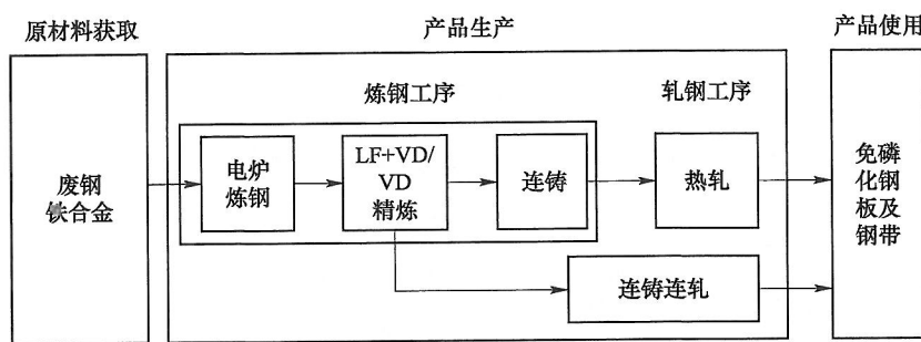
图 A.2 家具用免磷化钢板及钢带生命周期系统边界示意图(短流程)
