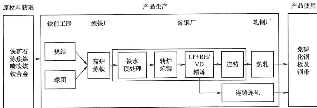
图 A.1 家具用免磷化钢板及钢带生命周期系统边界示意图(长流程)
