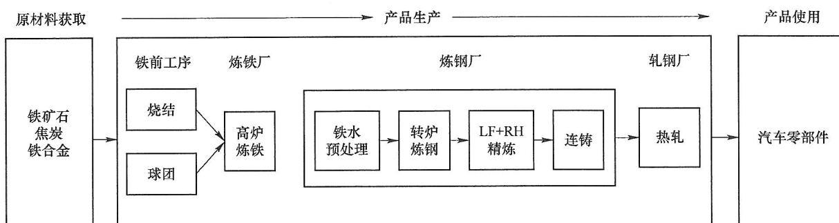
图 A.1 汽车用热轧高强度钢板及钢带生命周期系统边界示意图
