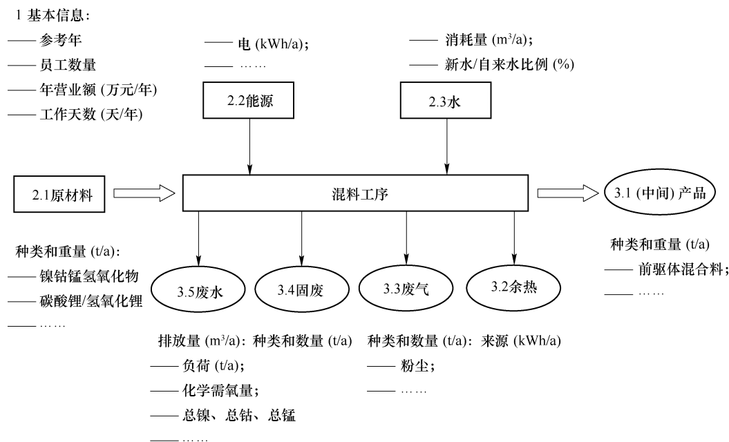
图 B.1 工序图
