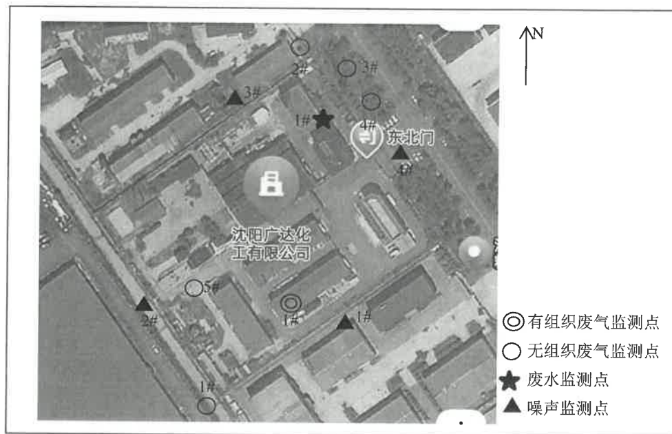
图 5-1 检测点位图
